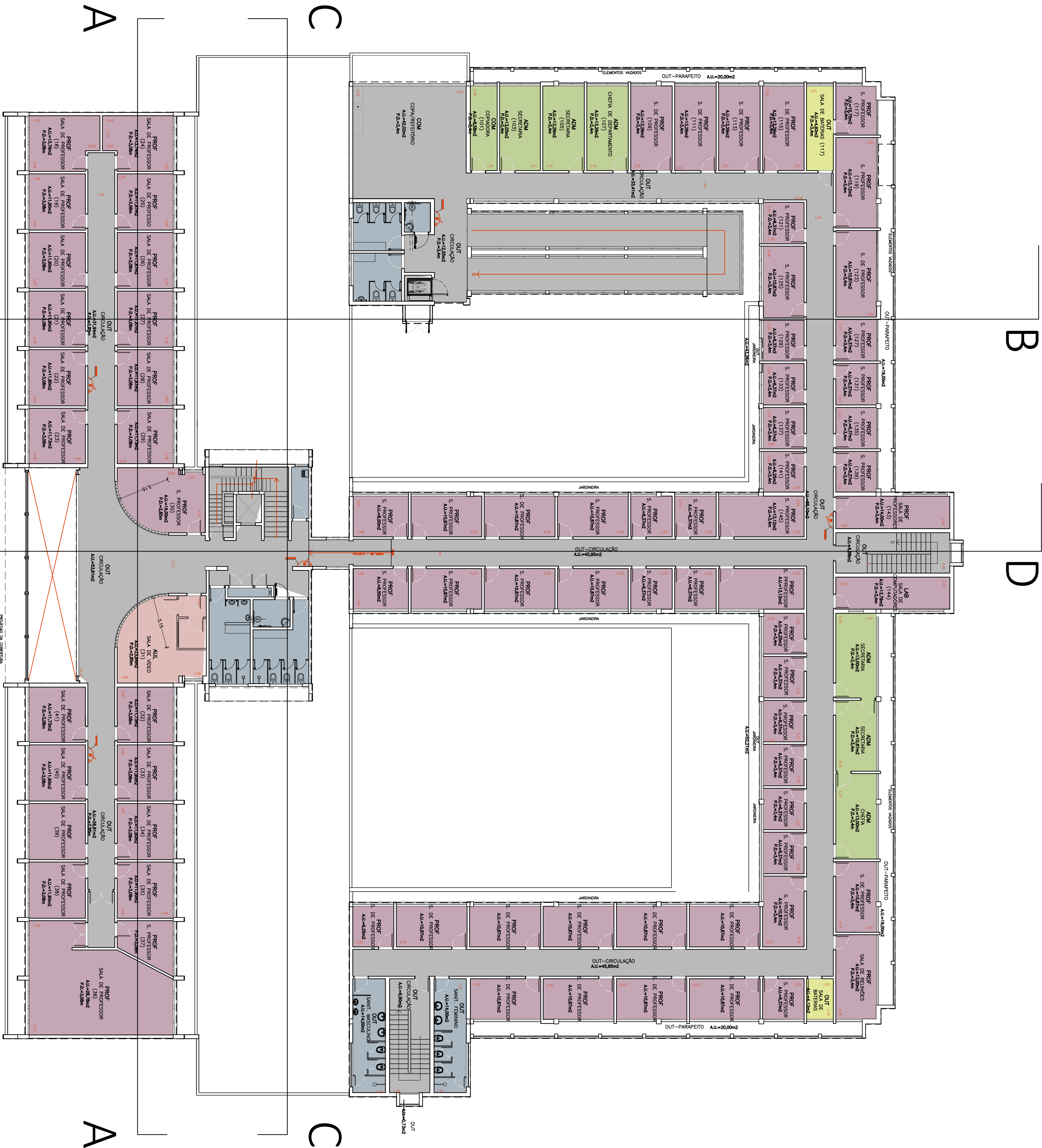
01 PLANTA - PAV. SUPERIOR 1:150 (m)
