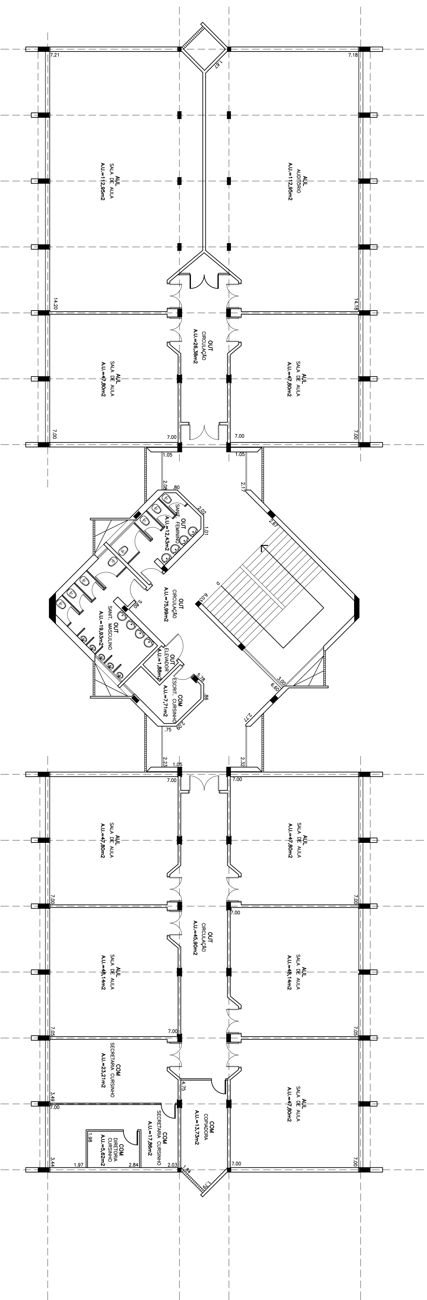
PLANTA PAVIMENTO SUPERIOR
